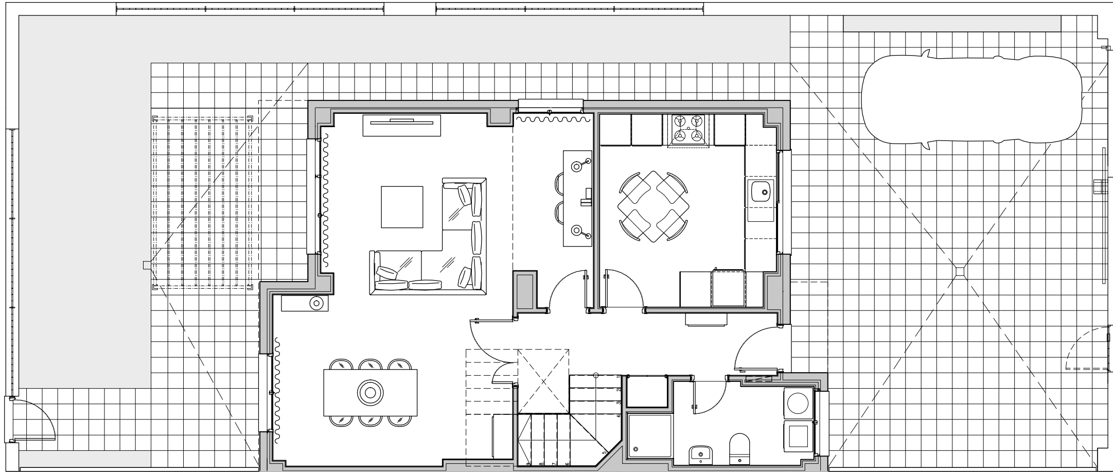
PLANTA BAJA
