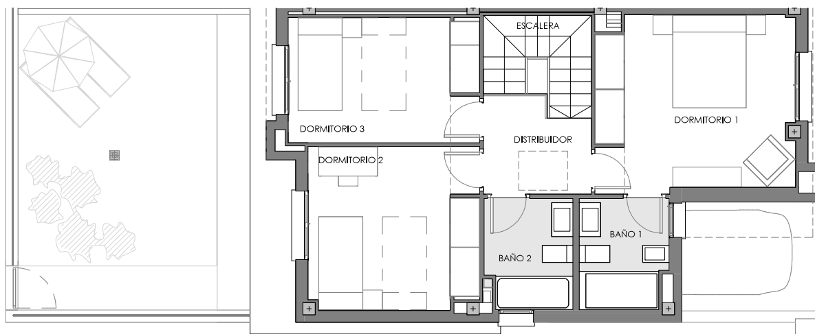
PLANTA PRIMERA
